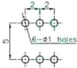
PCB Layout(Pattern Side)
