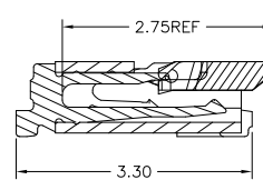
Section A-A Scale 2:1
