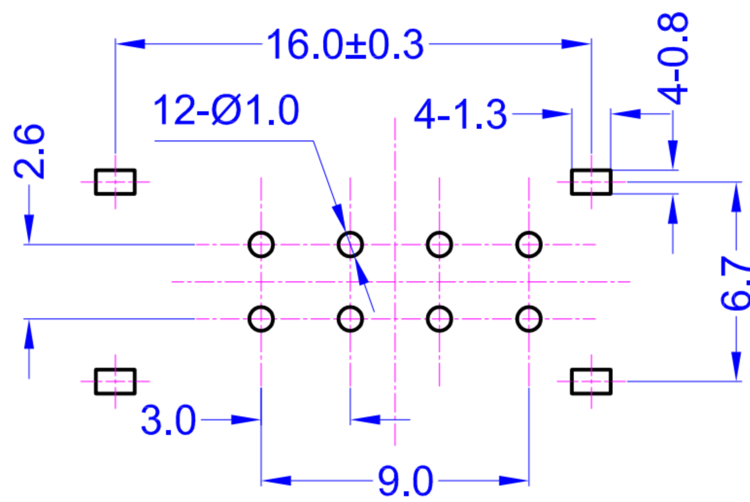
P.C.B LAYOUT
