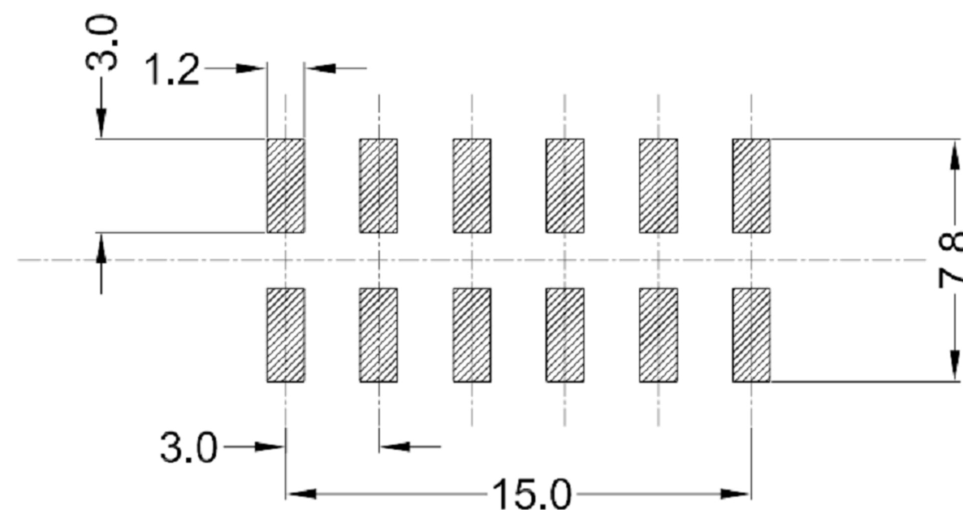
P.C.B LAYOUT
