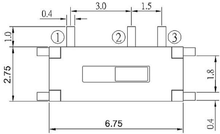
P.C.B LAND PATTERN
