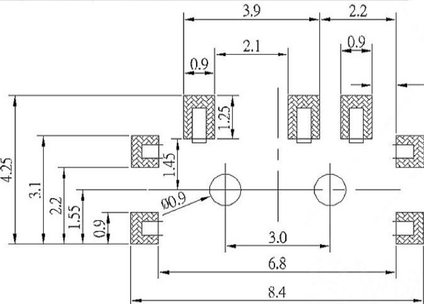
P.C.B LAND PATTERN
