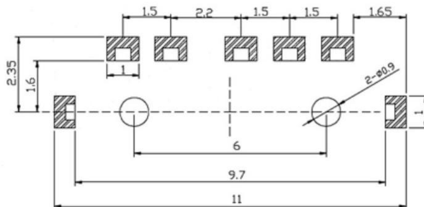
P.C.B layout
