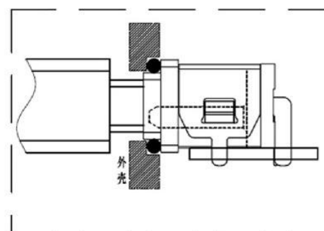
组装示意图
