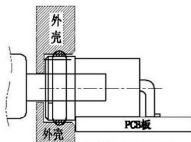
组装示意图
