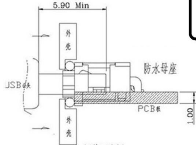
组装示意图
