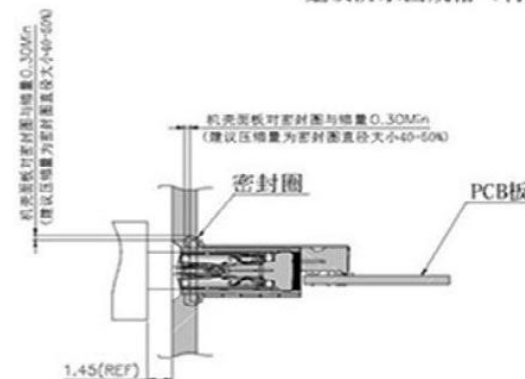
建议防水圈规格 (材质硅橡胶)
