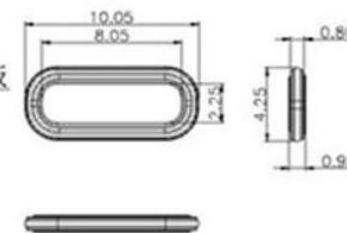
建议防水圈规格 (材质硅橡胶)
