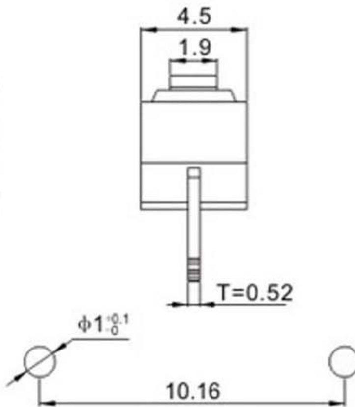
P.C.B Layout
