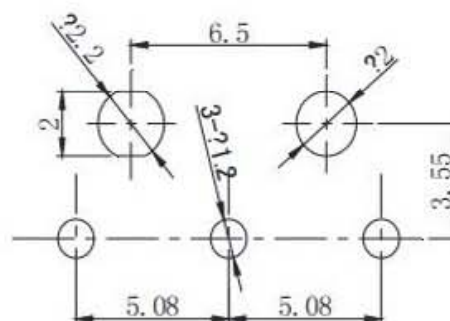
右側面PCB HOLE
