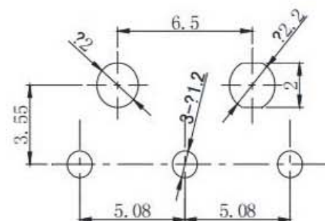
左側面PCB HOLE
