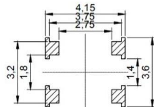
安装参考图
