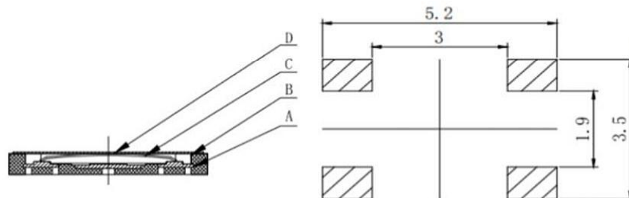
安装参考图
