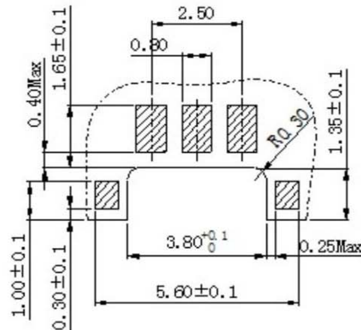
P.C.B LAND DIMENSION
