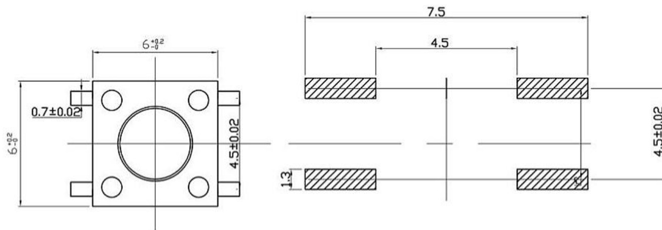
P.C.B. Land Pattern
