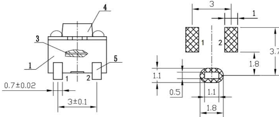
安装尺寸 (从焊锡面看)
