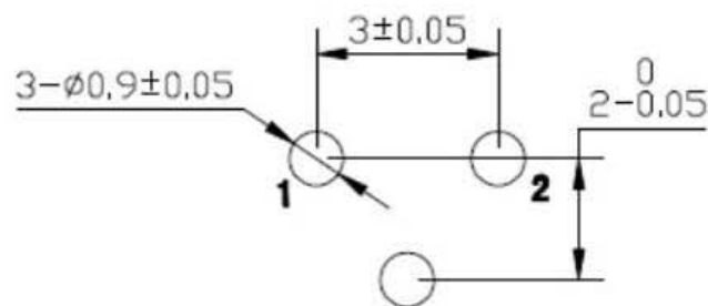
安装尺寸 (从焊锡面看)
