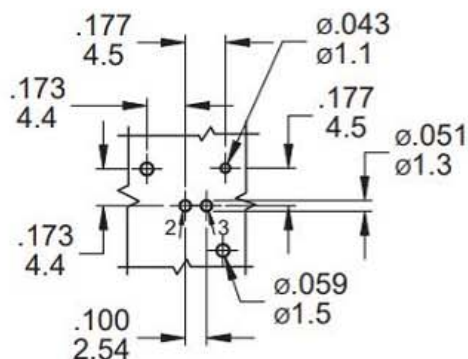
SPST
