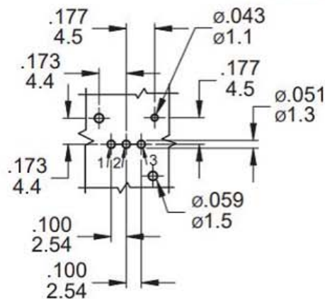
SPDT
