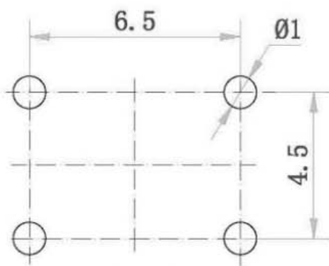
PCB板开孔尺寸(±0.1)
