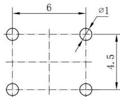
PCB板开孔尺寸(±0.1)
