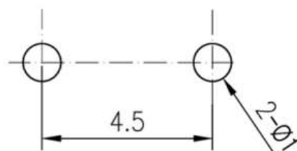
PCB线路板安装图(±0.1)
