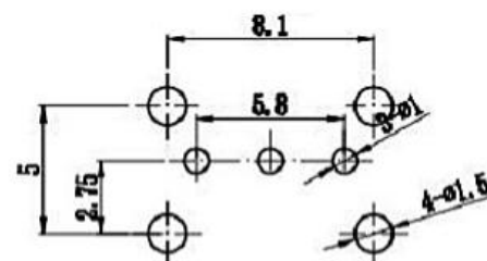
PCB线路板安装图(±0.1)
