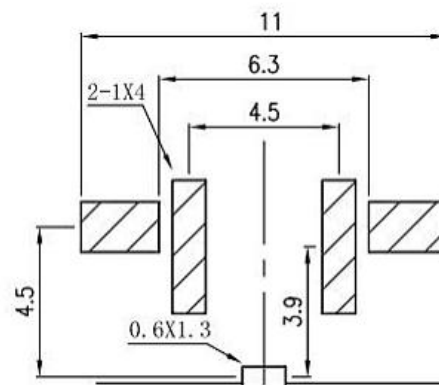
PCB线路板安装图(±0.1)
