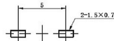
PCB线路板安装图(±0.2)
