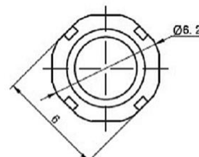
PCB线路板安装图(±0.2)
