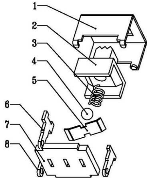
产品结构示意图
