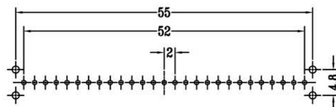
P.C.B LAYOUT
