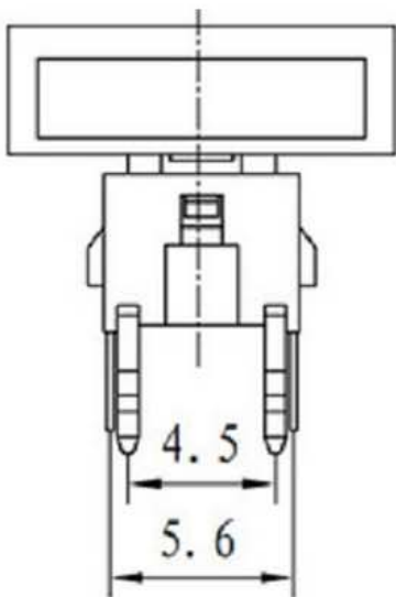
线路板安装孔图 P. C. B. Land Pattern
