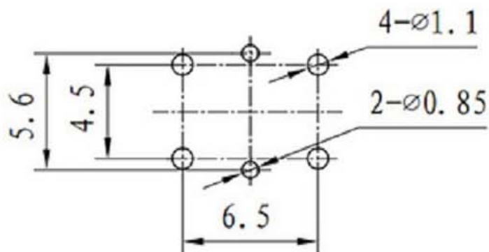
线路板安装孔图 P. C. B. Land Pattern
