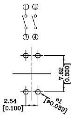
P.C.B LAYOUT
