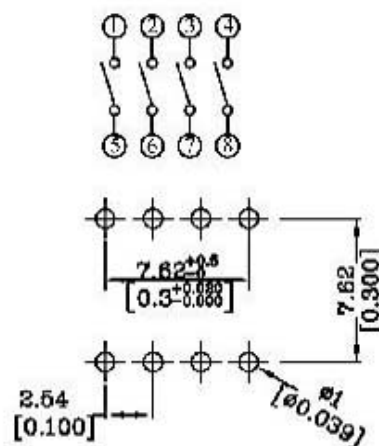
P.C.B LAYOUT
