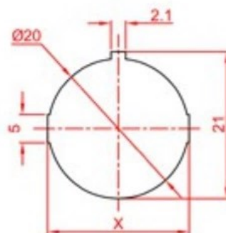
开孔尺寸
