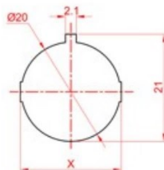
开孔尺寸
