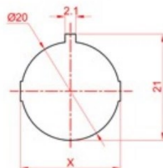
开孔尺寸
