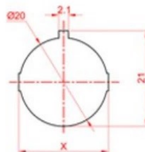
开孔尺寸
