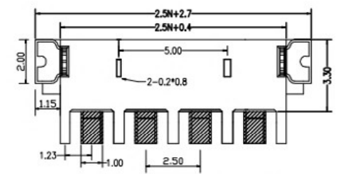
PCB LAYOUT(4pin)
