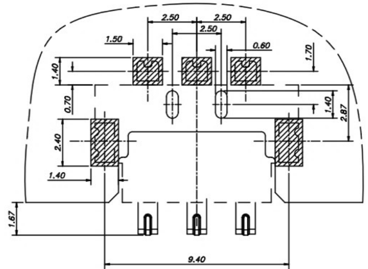
PCB布线图 未注尺寸公差: \pm 0.05
