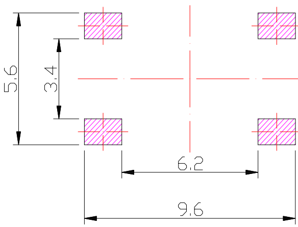
P.C.B LAYOUT
