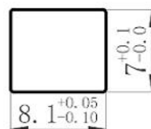
安装孔尺寸
