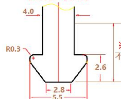
锁舌参考尺寸
