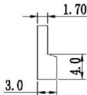
锁舌参考尺寸
