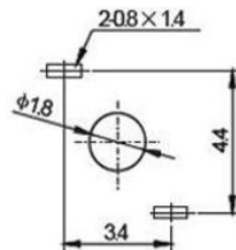
P. C. B开孔图
