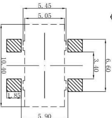
PCB 焊接尺寸图
