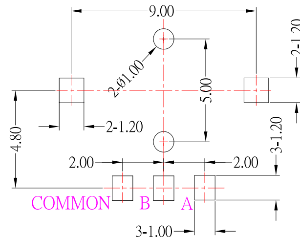
P.C.B LAYOUT
