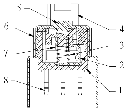
A - A
