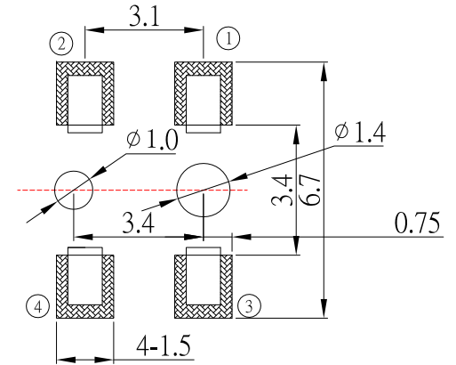
P.C.B LAYOUT
