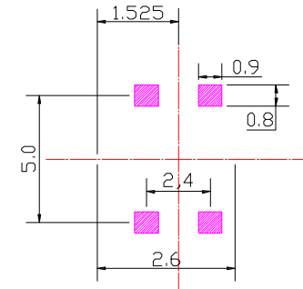
P.C.B LAYOUT
