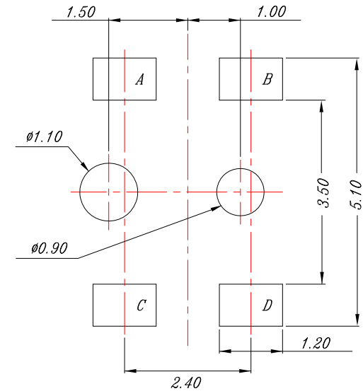
P.C.B LAYOUT
