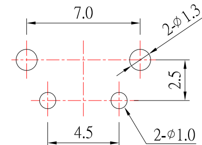
P.C.B LAY OUT
