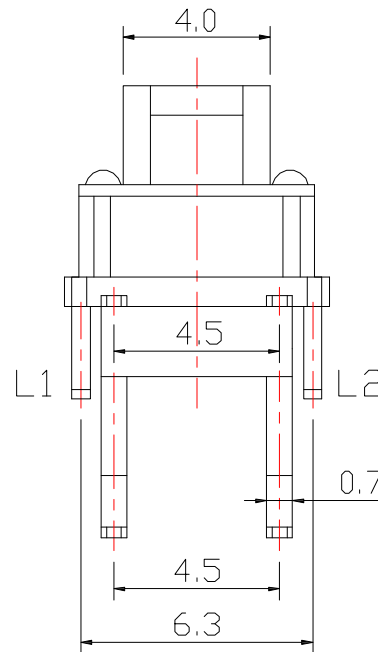
P.C.B LAYOUT
