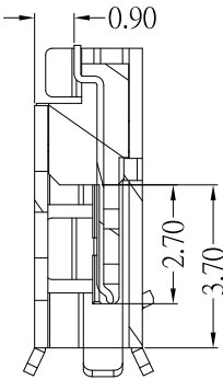
剖面 A-A
