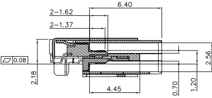
SECTION E-E SCALE: 1:1
